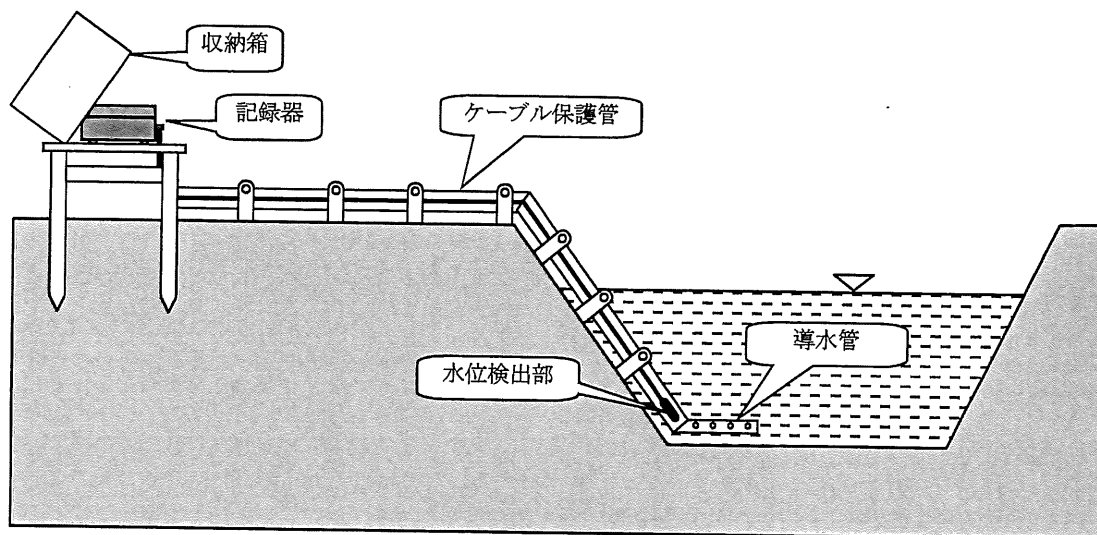
図 5.2 河川水位計設置方法
