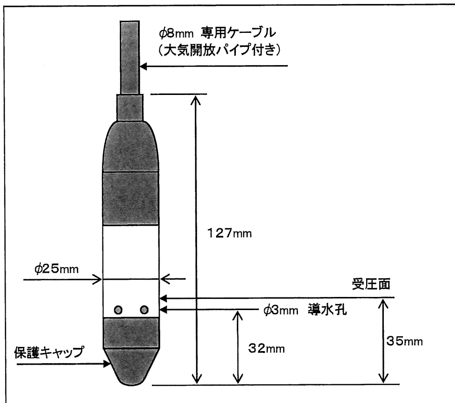
図 4.1 形状寸法図
