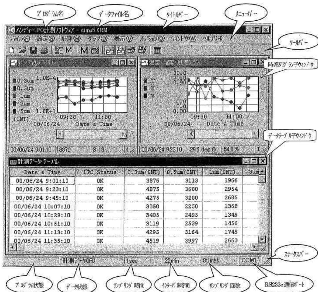
図5. 基本画面
