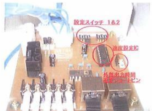
⑤電源スイッチと設定スイッチの位置
