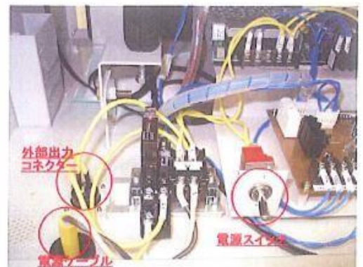
④電源ケーブルとコネクタの位置
