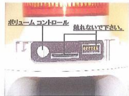
⑧前面パネルを外した状態
