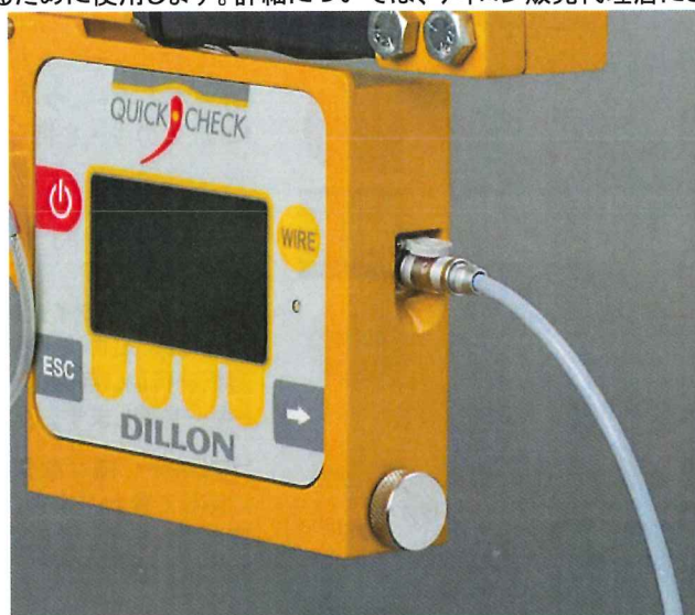
図 2.3 クイックチェックコネクタ
