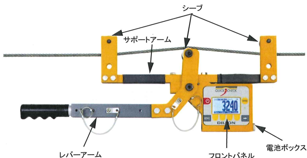
図 2.1 クイックチェックの部品
