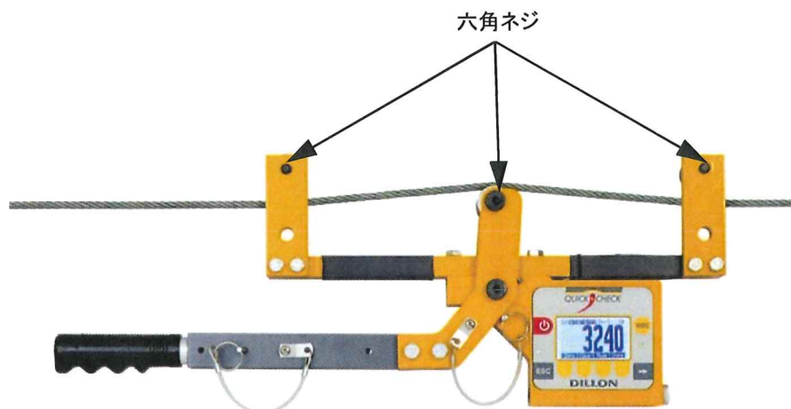
図 5.1 シーブの交換
