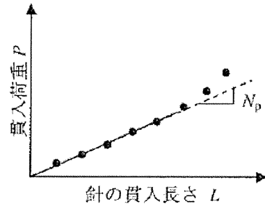
針貫入勾配の求め方 ( 机上型 )
