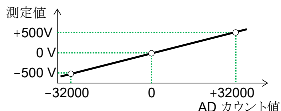
AD カウント値と測定値の関係
