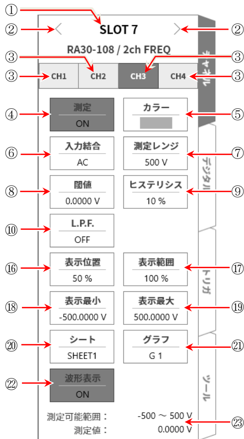
<入力電圧設定パネル>
