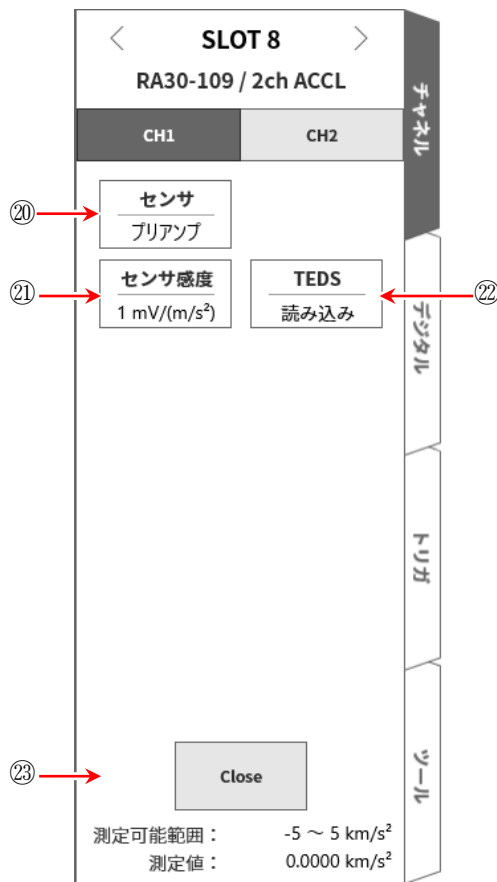
<センサ「プリアンプ」選択時>
