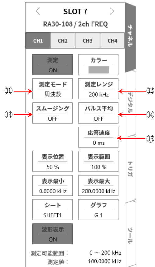
<測定モード設定パネル>
