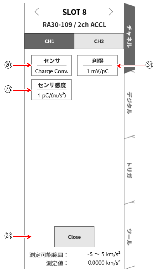
<センサ「Charge Conv.」選択時>
