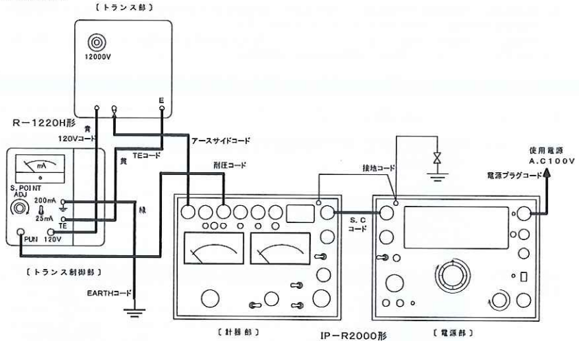
試験器結線図
