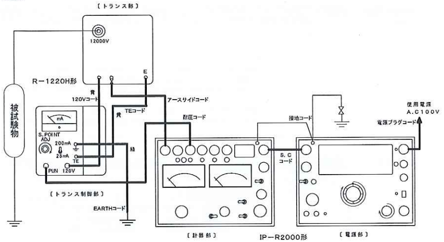
図2 絶縁耐力試験
