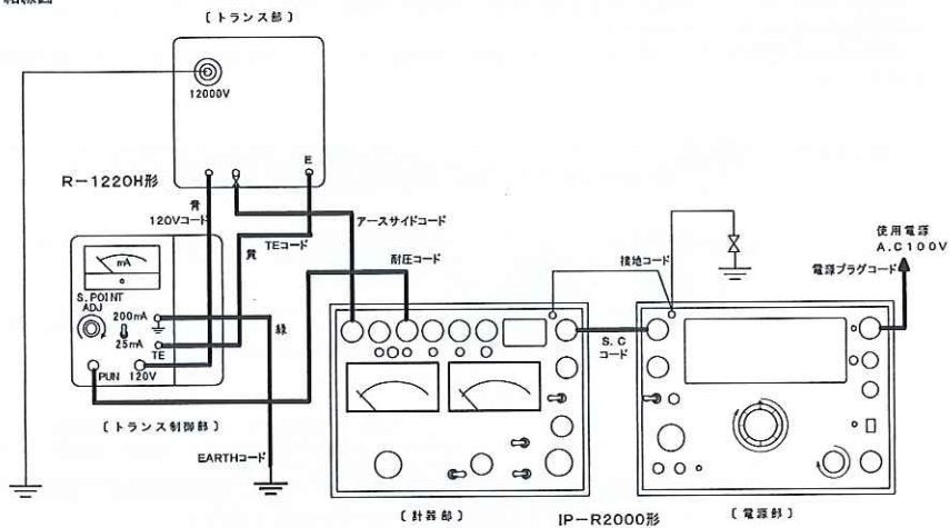
図1 遮断電流の設定
