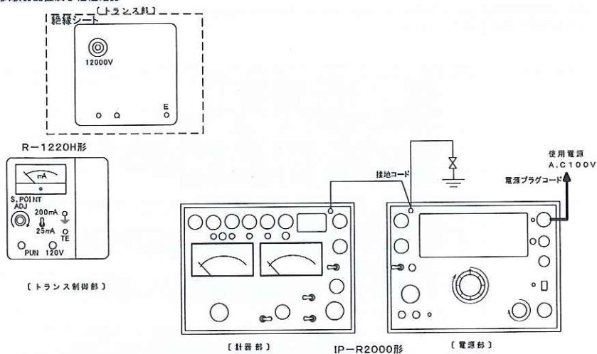
図1 試験器配置及び極性確認
