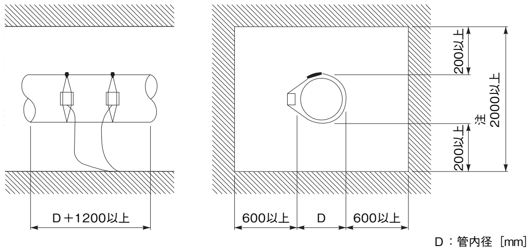
検出器取付け場所の必要スペース
