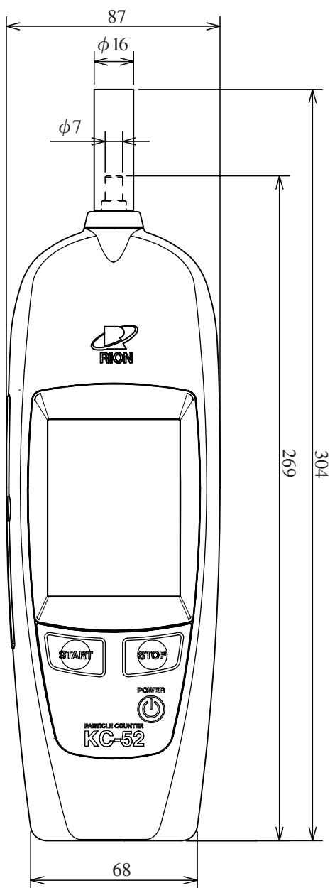
正面図
