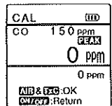
〈スパン調整画面〉
