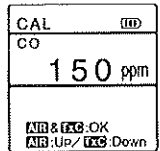
〈濃度設定画面〉
