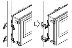
図 1: 単管クランプによる固定
