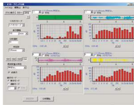
オクターブバンド分析画面例
