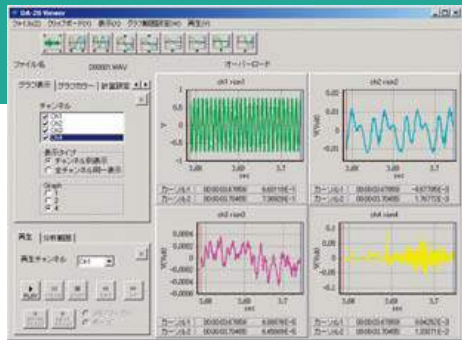
4ch表示画面例
