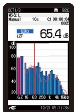
重ね合わせ分析画面
