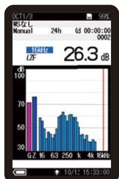
1/3オクターブ分析画面(高域)
