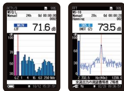
1/3オクターブ分析表示(低域)
