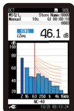
NC曲線表示画面
