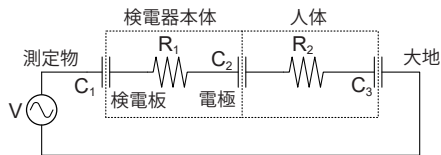
等価回路
