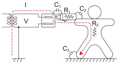
測定原理図
