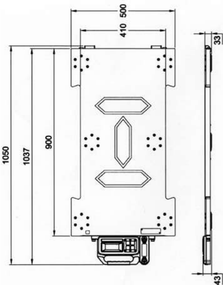
計量台
