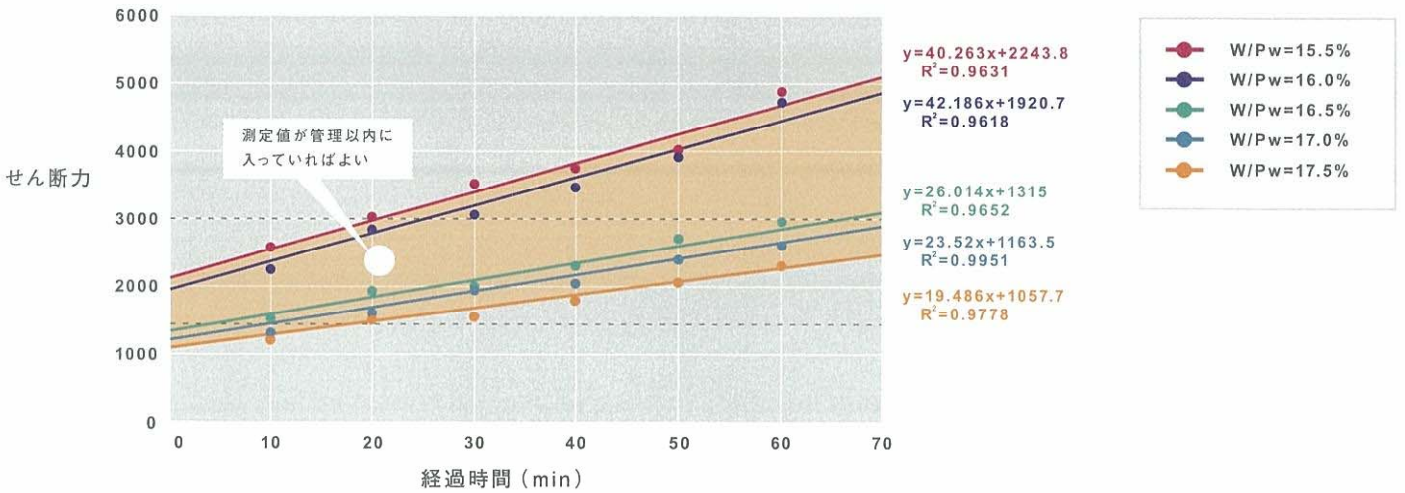
経過時間とせん断力の関係
