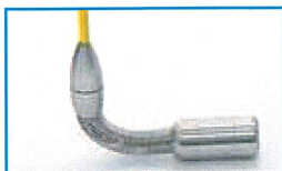
曲げる事の出来る最小半径は 90 度の直 角配管で 50mm 幅があれば進めます。
