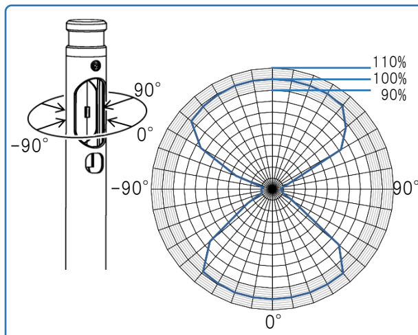
風速の指向特性(水平方向)
