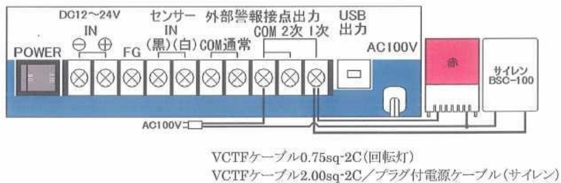
5-6 サイレンと回転灯を同じ警報で作動するように接続する例
