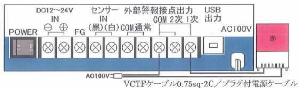
5-5 外部接点出力と回転灯の接続例
